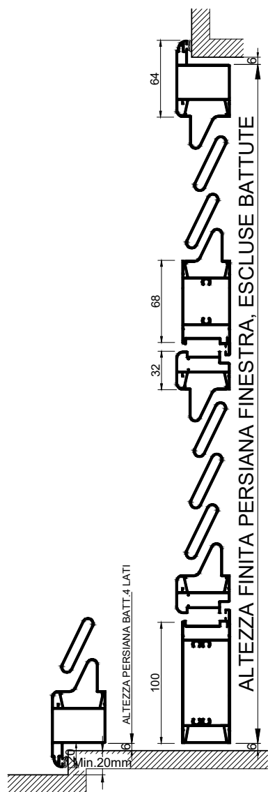
ANTA GIRO TAGLIO 45° (NO ZOCCOLO)
