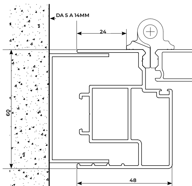
TELAIO TELESCOPICO CON COMPENSATORE A MURO
