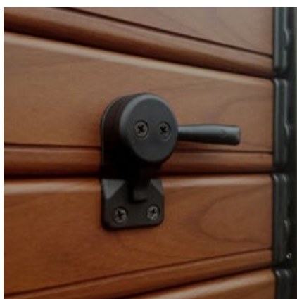
MANIGLIETTA MINILEVA PER ORIENTABILI IN CASO DI ANTE SCORREVOLI, A LIBRO OPPURE DI SPAZI RIDOTTI.
