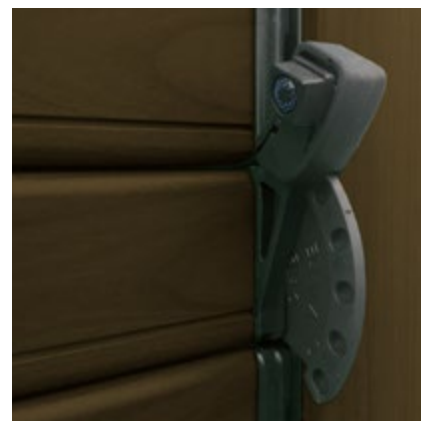
MANIGLIETTA PER LAMELLE ORIENTABILI STANDARD.
