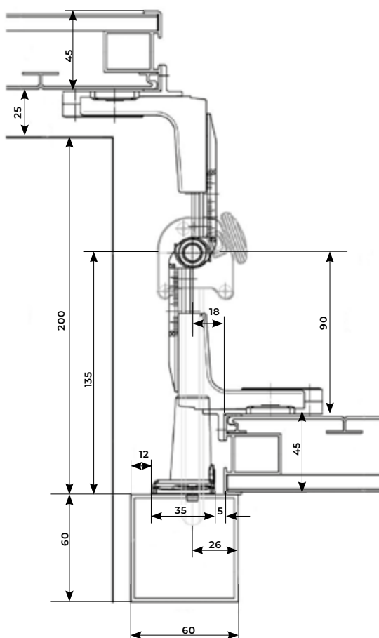
ESEMPIO CON SPALLETTA MASSIMA 26CM CON TELAIO 60x60 MASSIMA 24CM CON TELAIO 60x40
