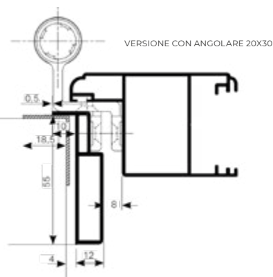
TELAIO TZS 2 ANTE PORTAFINESTRA
