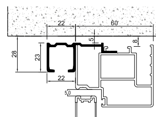
TELAIO CON BINARIO PER GRANDI LUCI
