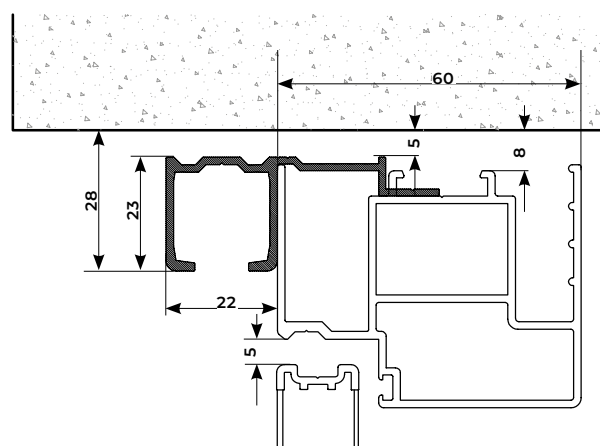
TELAIO CON BINARIO PER GRANDI LUCI
