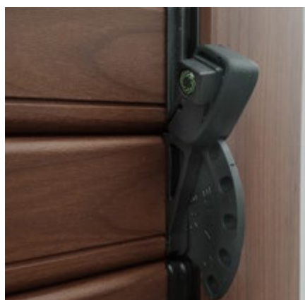
DETTAGLIO MANIGLIETTA PER LAMELLE ORIENTABILI STANDARD.
