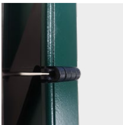
DETTAGLIO CERNIERA A SNODO PER SPORTELLO APRIBILE.
