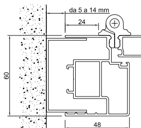
TELAIO TELESOPICO CON COMPENSATORE A MURO
