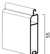
in allum. 55 mm Terminale 13X55 Universale
