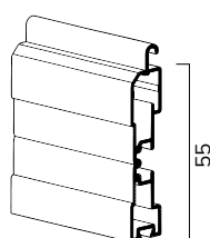
in allum. 55 mm Terminale 12X55
