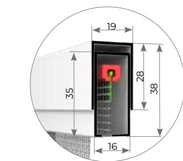
DETTAGLIO GUIDA SUPERIORE
