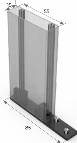
TUBOLARE 55 x 15
