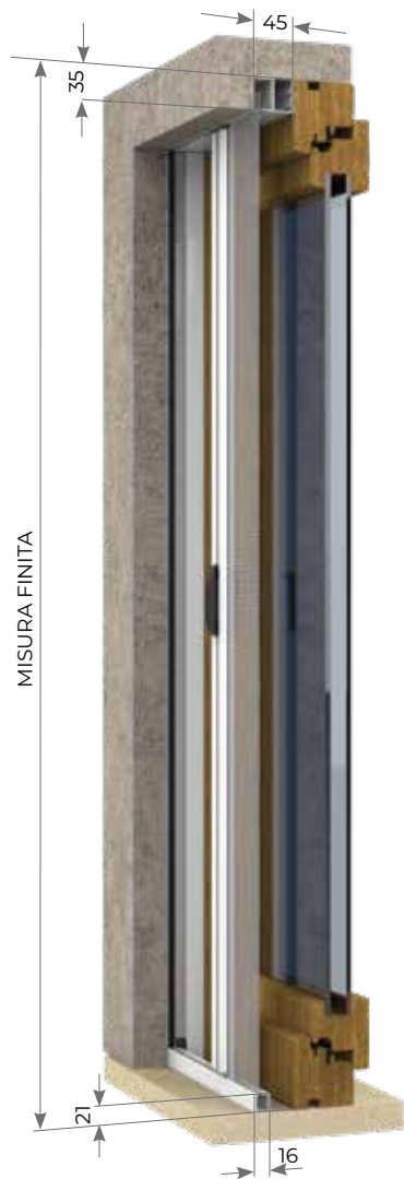
OPTIONAL ACPL0139 STAFFA AD U PER FISSAGGIO LATERALE | FIS. GUIDA SUPERIORE - GUIDA 45X35
