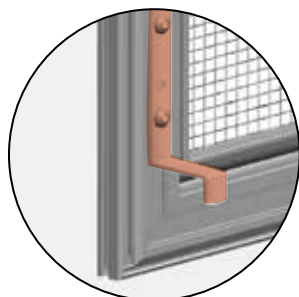
CLIP A "Z" misure disponibili min. 6mm - max 30mm
