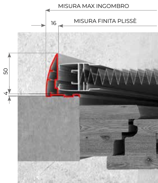
FISSAGGIO FRONTALE PLISSÈ ZERO
