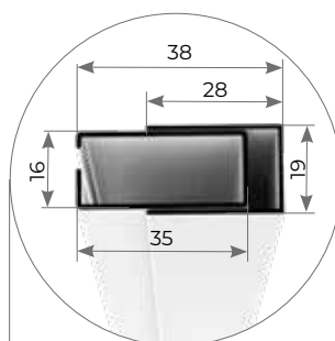
GUIDA TELESCOPICA
