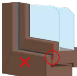
FINESTRE IN LEGNO CON ROMPI GOCCIA SUL TELAIO O ANTA COMPLANARE
