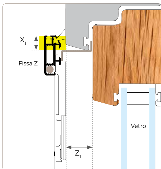
CLIP A "Z" misure disponibili min. 6mm - max 30mm
