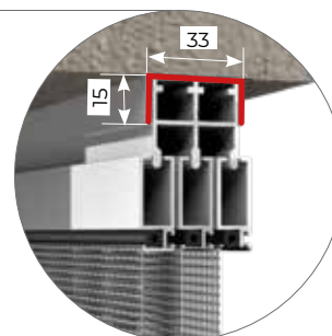
CON KIT DI COMPENSAZIONE 3 ANTE
