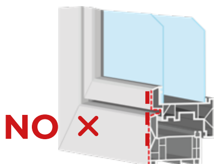
FINESTRE IN PVC O ALLUMINIO CON ANTA E TELAIO COMPLANARI
