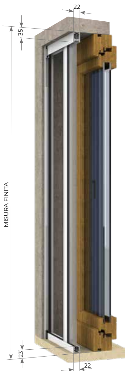
PROFILO RINFORZO MANIGLIA LATERALE
