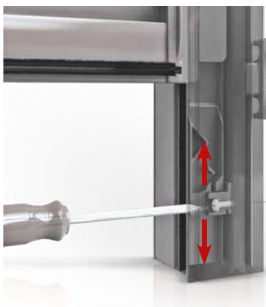
CLIC CLAC AGGANCIO REGOLABILE
