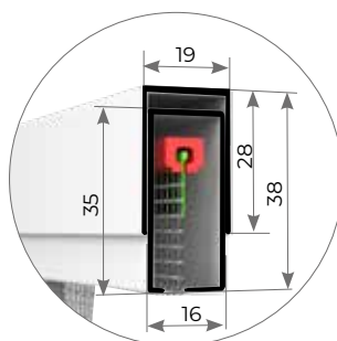
DETAGLIO GUIDA SUPERIORE
